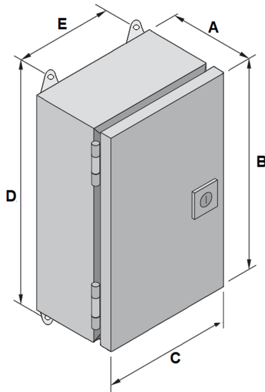
TC16 Dimensions
